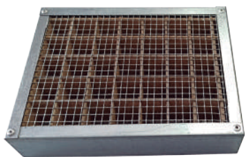
Rejilla intumescente EI2-60
